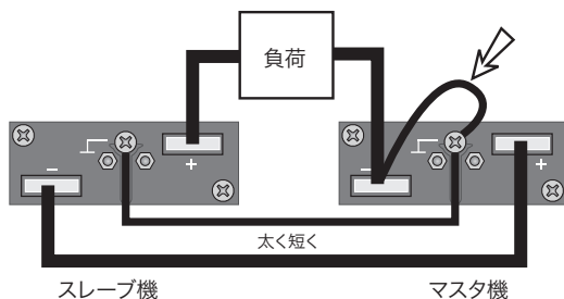
図 5-3 直列運転の負荷接続 (マスタ機の－端子をシャシ端子へ接続する例)
