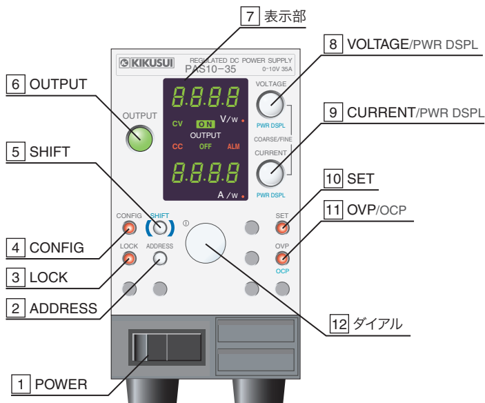
図 6-1 前面パネル（例：350 W タイプ）
