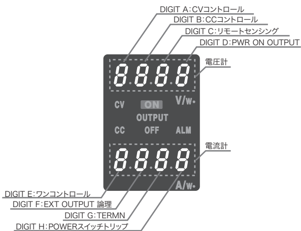
図 3-2 CONFIG 表示
