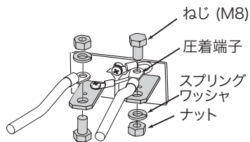
図 3-4 M8 ねじによる接続
