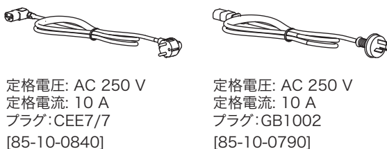
図 1-4 別売の 3 極プラグ付き電源コード
