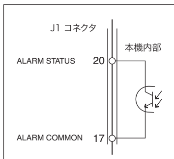
図 2-9 ALARM 信号
