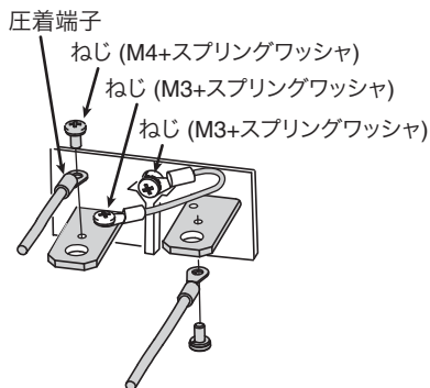
図 3-3 M4 ねじによる接続
