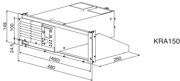
☒ P-1 ラックマウントフレーム
