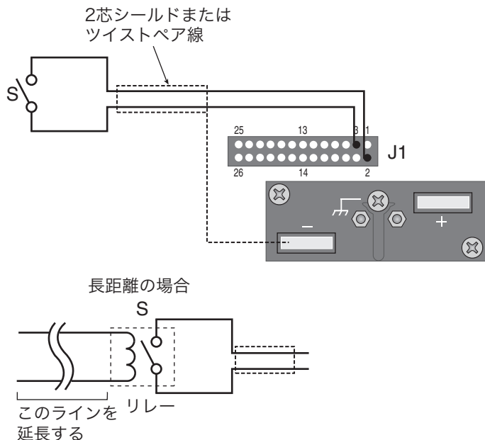
図 4-7 ON/OFF コントロールの接続
