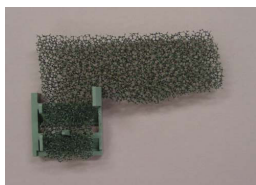
図 7-2 ダストフィルタの取り付け
