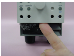
図 7-4 フィルタのセット
