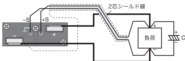
図 3-5 リモートセンシングの接続
