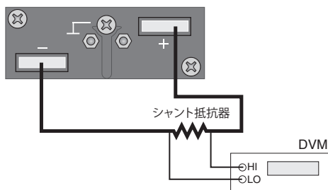
図 7-16 電流系校正の接続
