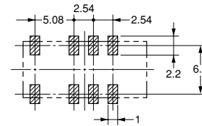
プリント基板加工寸法 (TOP VIEW) 寸法公差は±0.1mmです。
