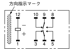
端子配置/内部接続図 (TOP VIEW)
