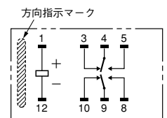
端子配置/内部接続図 (BOTTOM VIEW)
